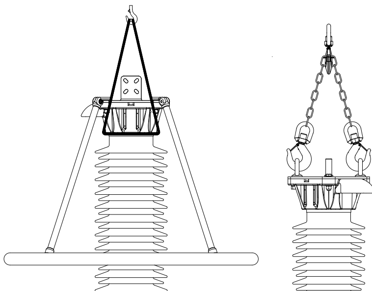
Abb.3.1 Anhebungsmöglichkeiten
